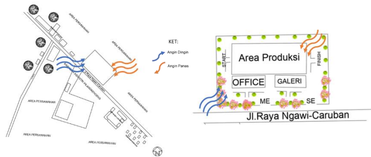
Gambar 4. Analisa angin
