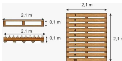
Gambar 2 Palet Kayu Untuk Alas Drum (Sumber: Desain Penmelitian,2019)
