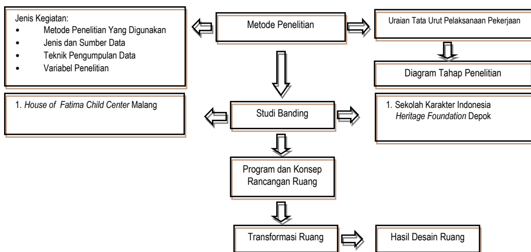
Diagram 1 Alur Perancangan
