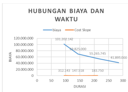
Gambar 4. Perbandingan hubungan biaya dan waktu Pengerjaan Proyek Pada Lintasan Kritis Proyek Pembangunan Kapal Cargo RO-PAX 300.
