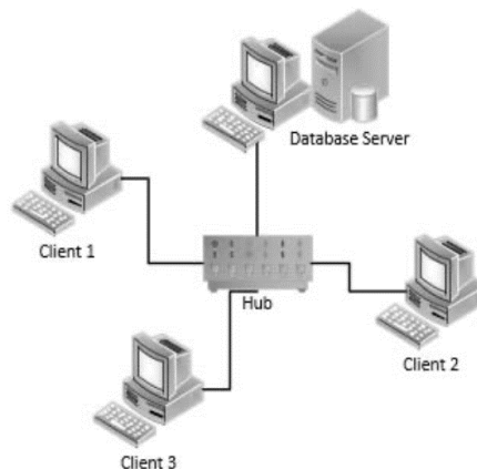
Gambar 1. Arsitektur Client-Server
