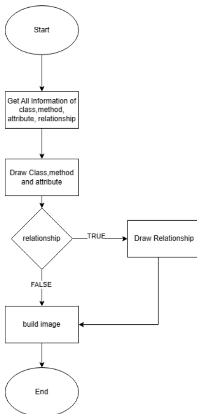
Gambar 4. Proses penggambaran class diagram
