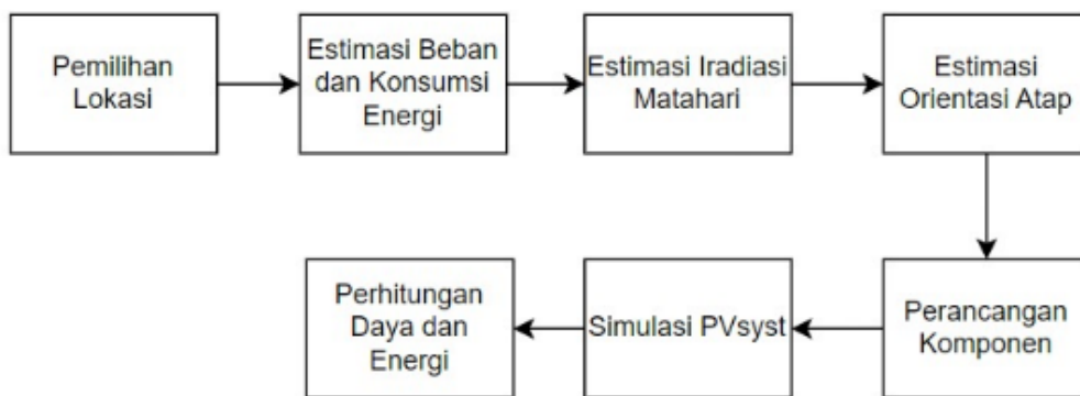
Gambar 1. Metodologi Penelitian
