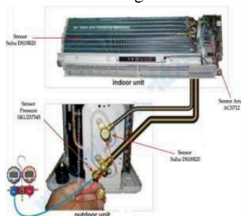
Gambar 1. Perancangan Hardware
