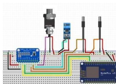
Gambar 2. Rangkaian Sistem Monitoring AC berbasis IoT dengan ESP8266
