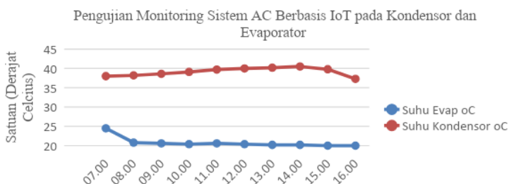
Gambar 6. Grafik Pengujian Monitoring Sistem AC Berbasis IoT pada Kondensor dan Evaporator
