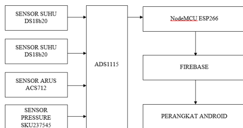
Gambar 3. Blok Diagram Sistem
