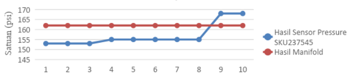
Grafik Perbandingan Hasil Pengujian Sensor Pressure SKU237545 Dengan Manifold
