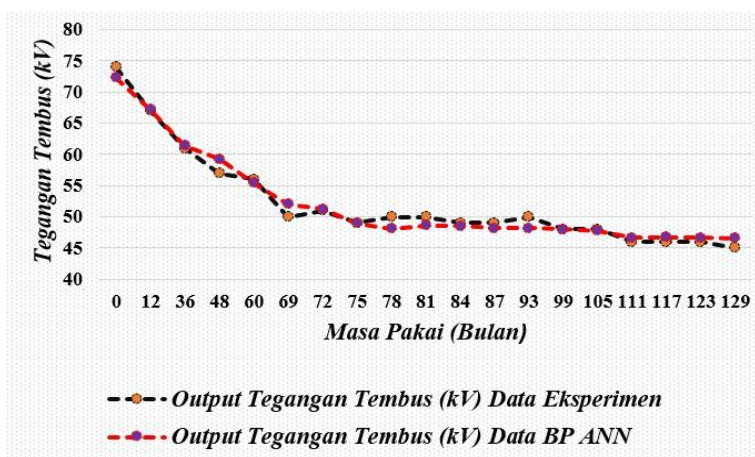
Gambar 4. Grafik Perbandingan Data Eksperimen dan ANN
