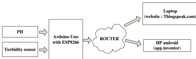
Gambar 1. Blok Diagram Perancangan Sistem
