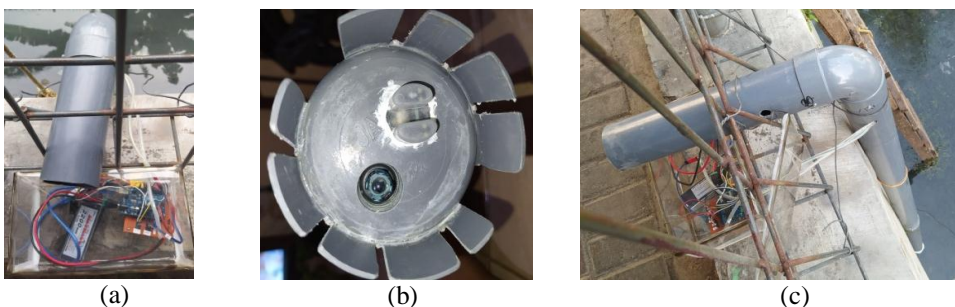
Gambar 4. a) komponen pada akrilik, b) komponen pada pipa paralon, c) pemasangan hardware di lapangan
