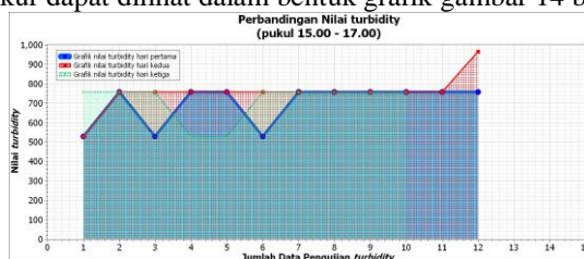
Gambar 14. grafik nilai Turbidity pukul 15.00 – 17.00
