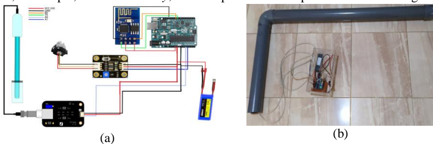
Gambar 3. a) desain wiring hardware , b) desain hardware
