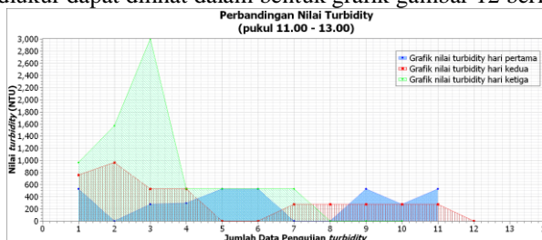
Gambar 12. grafik nilai Turbidity pukul 11.00 – 13.00
