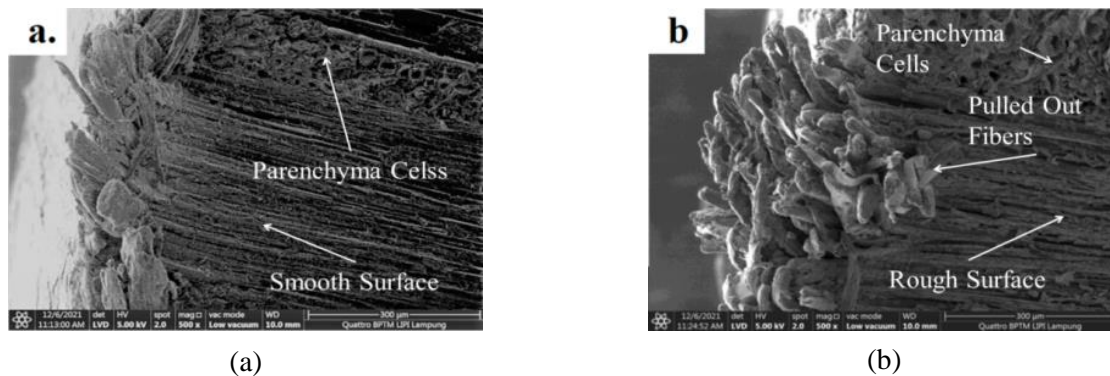
Gambar 8. Hasil uji fraktografi SEM pada permukaan buku bambu betung dengan perbesaran 500X (a) tanpa perlakuan NaOH (b) dengan perlakuan NaOH 5%.
