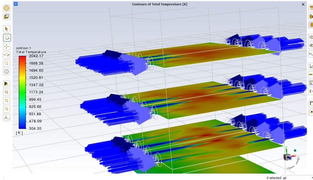
Gambar 6. Kontur temperatur (K) pada inlet batubara dan udara
