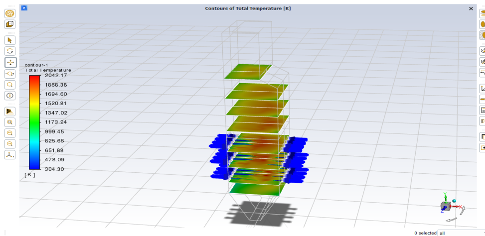
Gambar 5. Kontur temperatur (K) pada furnace
