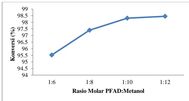
Gambar 4. Hubungan Rasio Molar terhadap Konversi PFAD.
