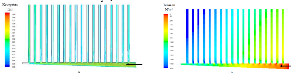
Gambar 6. Iso-surface (a) Pathline Kecepatan, dan (b) Kontur Tekanan pada inlet header trapezoidal blocker dengan Reynolds Number 5146.
