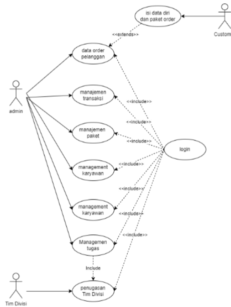
Gambar 3 Use Case Apikasi
