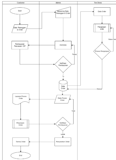
Gambar 2 Rancangan Sistem yang diusulkan
