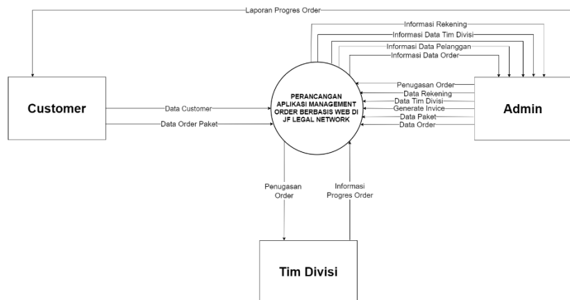
Gambar 5 Diagram Kontek Aplikasi
