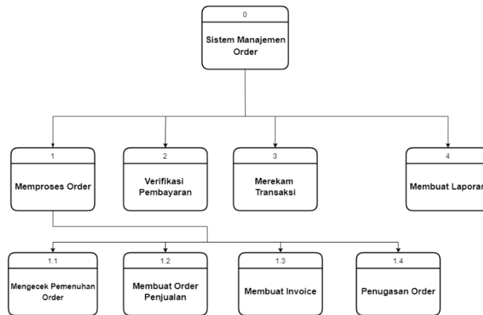
Gambar 4 Diagram Jenjang Aplikasi
