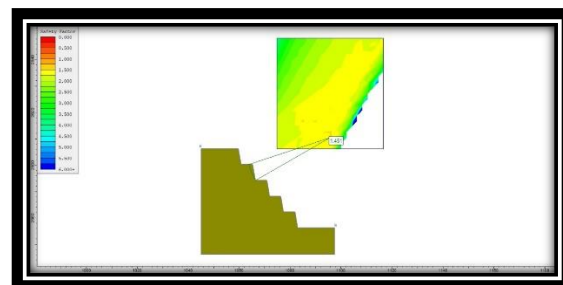
Gambar 9: Lereng Keseluruhan Tinggi 6 Meter D 0,7 adalah 1,451
