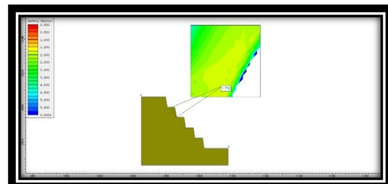
Gambar 8: Lereng Keseluruhan Tinggi 6 Meter D 0,5 adalah 1,770
