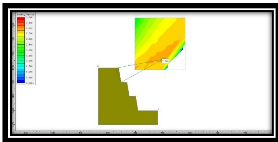
Gambar 13: Lereng Keseluruhan Tinggi 10 Meter D 0,7 adalah 1,124
