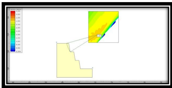
Gambar 12: Lereng Keseluruhan Tinggi 10 Meter D 0,5 adalah 1,357
