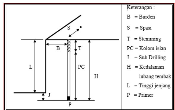
Gambar 1: Geometri Peledakan Menurut R.L. Ash, 1967
