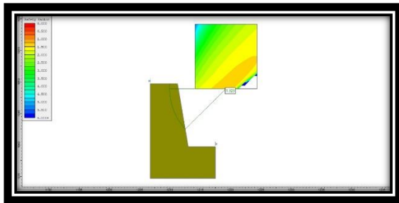
Gambar 11: Lereng Tunggal Tinggi 10 Meter D 0,7 adalah 1,323
