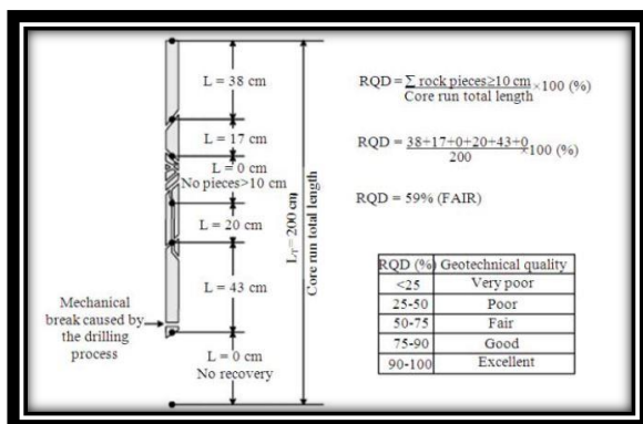
Gambar 3 : Prosedur Pengukuran RQD
