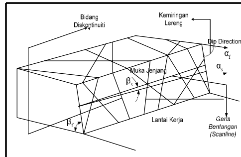
Gambar 4: Pengukuran Bidang Diskontinuiti dengan Metode Scanline (Kramadibrata, Suseno, 2002)
