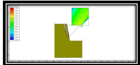
Gambar 6: Lereng Tunggal Tinggi 6 Meter D 0,5 adalah 1,940
