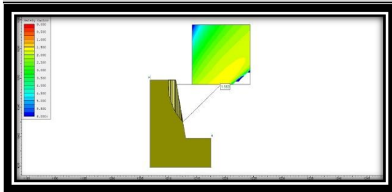
Gambar 10: Lereng Tunggal Tinggi 10 Meter D 0,5 adalah 1,563
