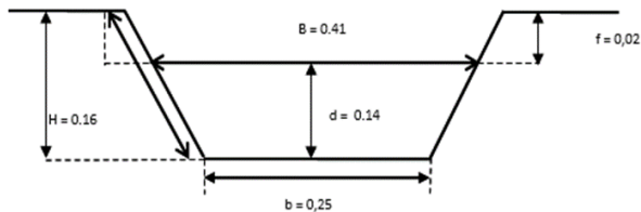
Gambar 5: Penampang Dimensi Saluran Drainase
