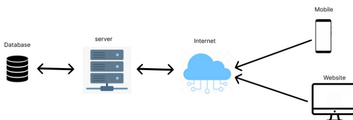
Gambar 1. Desain sistem
