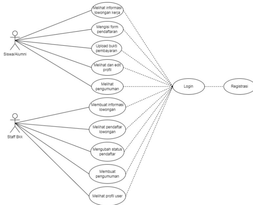
Gambar 2. Usecase sistem
