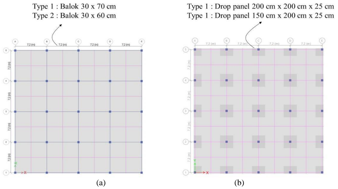
Gambar 3. Denah pemodelan struktur; (a) Pelat dengan balok, (b) Flat slab dengan drop panel
