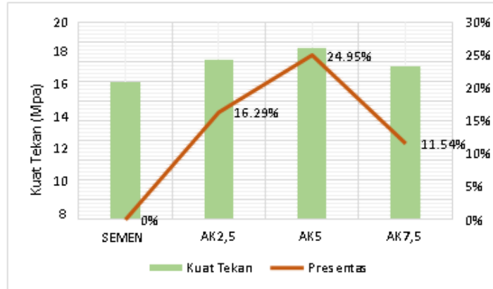
Gambar 4. Grafik Perbandingan Persentase Peningkatan Kuat Tekan Mortar Abu Kayu
