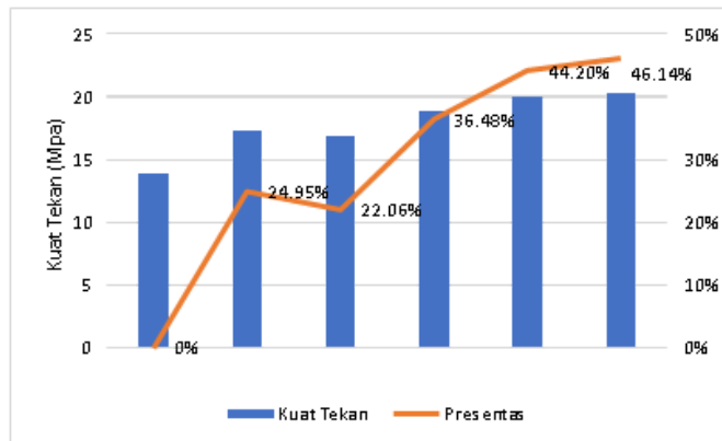
Gambar 5. Grafik Persentase Nilai Kuat Tekan Mortar Campuran Abu Kayu dan Fly Ash
