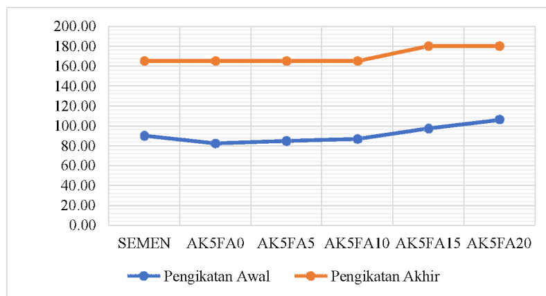
Gambar 3. Grafik Perbandingan Pengikatan Awal dan Akhir
