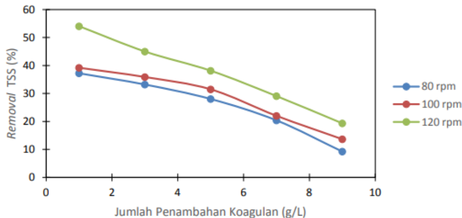
Gambar 4. Pengaruh Penambahan Koagulan terhadap Removal TSS
