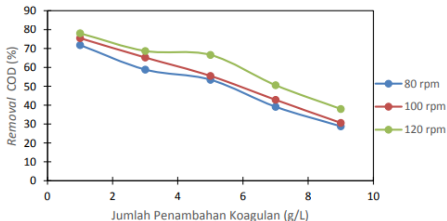
Gambar 3. Pengaruh Penambahan Koagulan terhadap Removal COD
