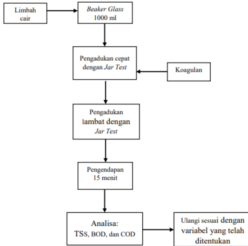
Gambar 1. Skema Proses Koagulasi-Flokulasi
