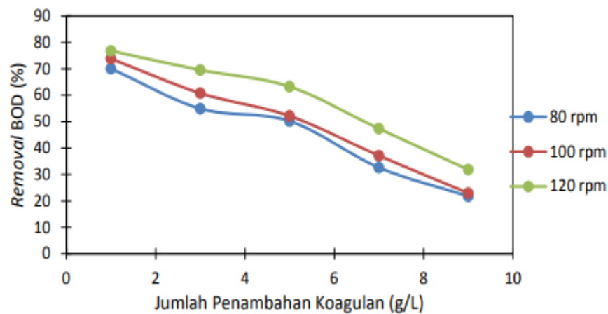
Gambar 2. Pengaruh Penambahan Koagulan terhadap Removal BOD
