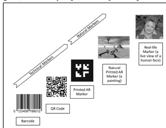
Gambar 1. Evolusi Marker.
