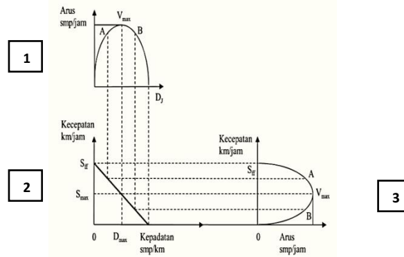
Gambar 1. Grafik Hubungan Volume, Kecepatan dan Kepadatan Sumber: Indrajaya, 2002., dalam Ariandi, dkk., 2016.
